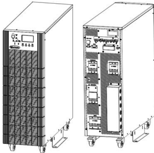
Рис.1-10 Внешний вид ИБП Легион-3Φ-20/30/40К-Ш/30/40К-С (без встроенных батарей)
