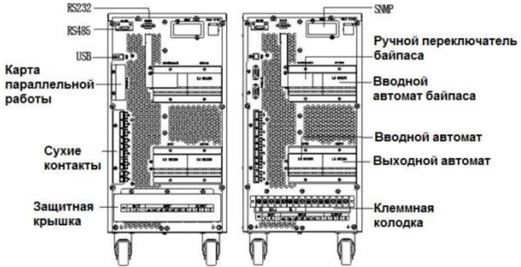
Рис.1-9 Компоновка ИБП Легион-3Φ-10К-Ш/15/20К-С, вид сзади
