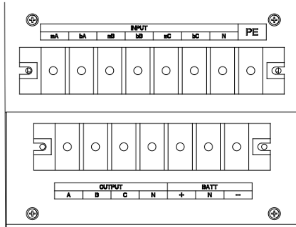
Рис. 2-13 Клеммная колодка на ИБП ЛЕГИОН-3Φ-40К-Ш
