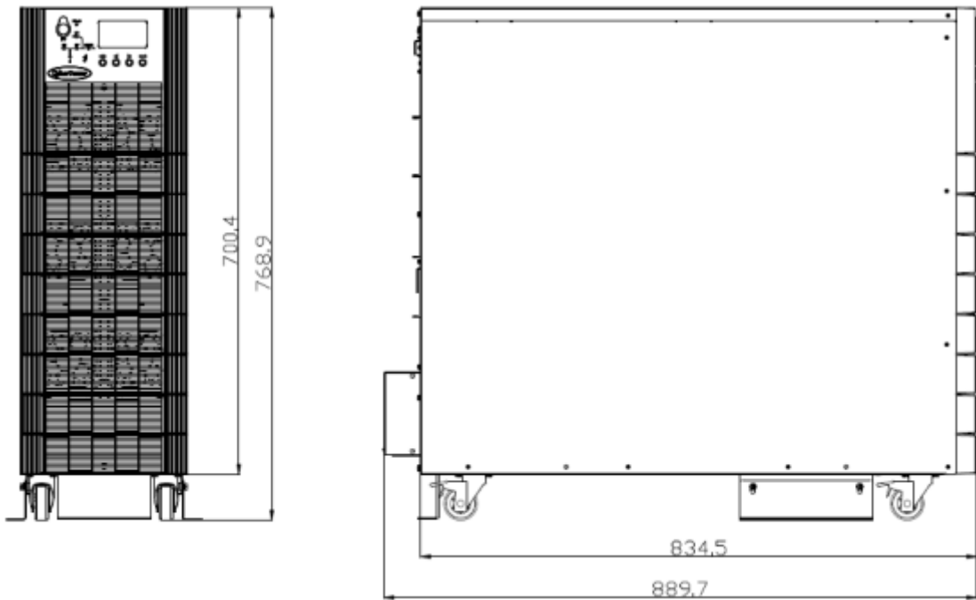
Рис.2-3 Габариты ЛЕГИОН-3Ф-40К-Ш (ед. изм.: мм)
